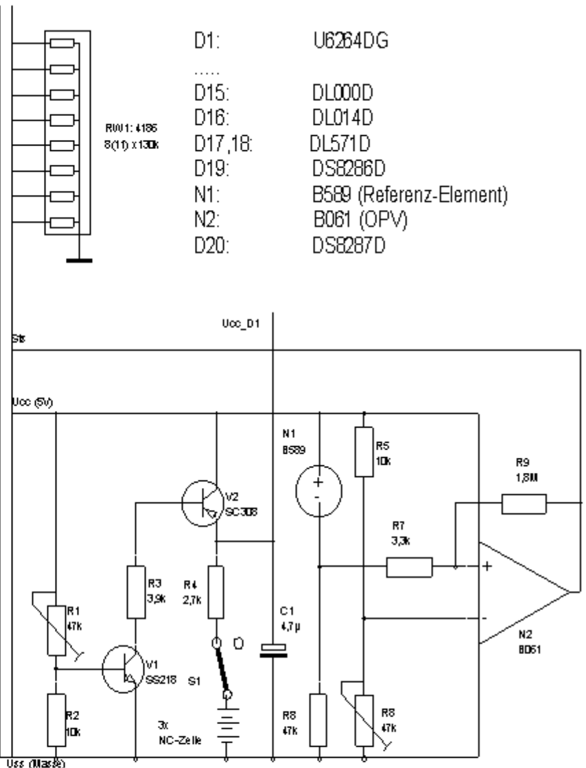
K1520-Anschluss - Batteriestützung Ergänzung zur BG 8k-DualPortRAM KC85/3-Zusatzgerät SEW
